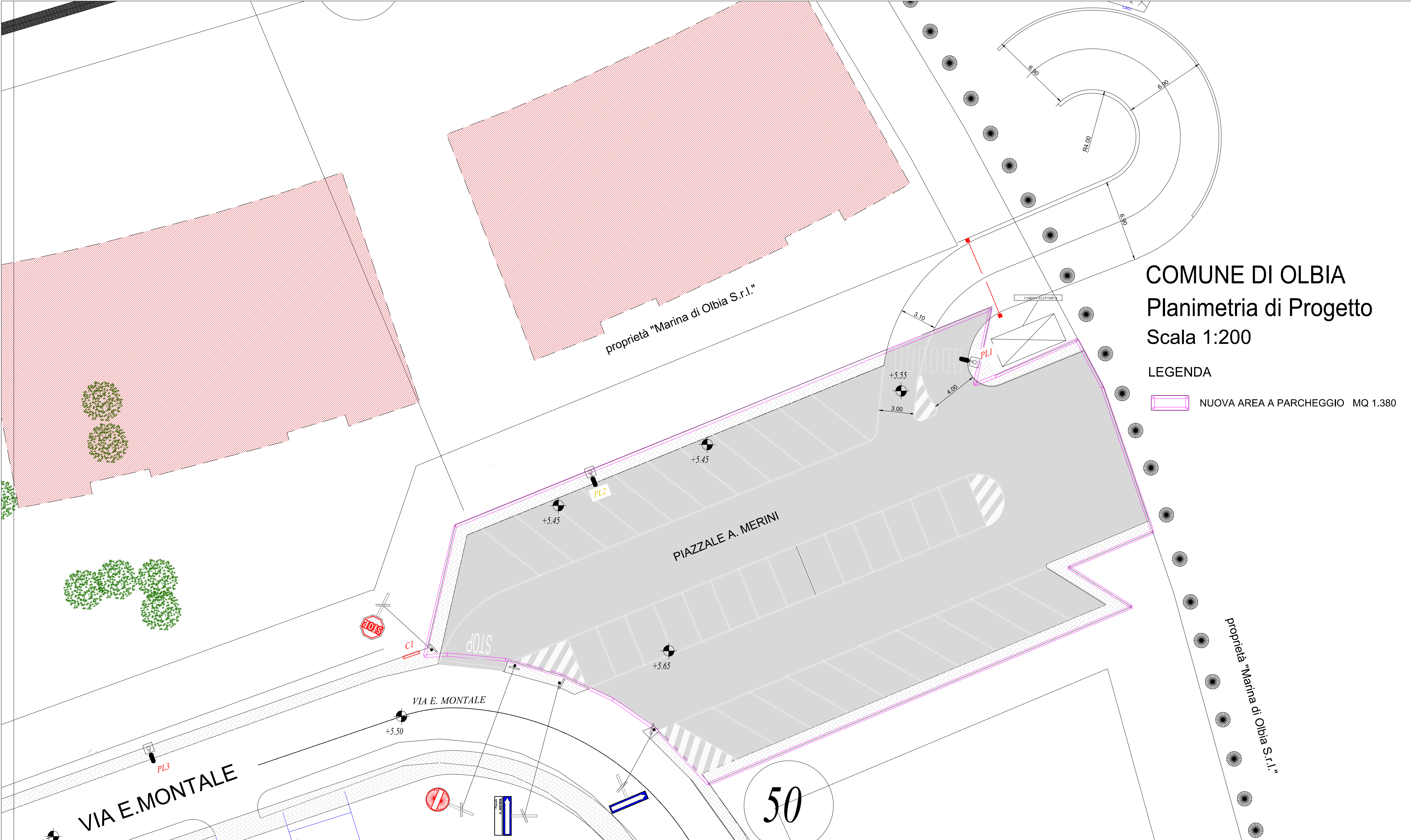
PLANIMETRIA TRATTO VIA MONTALE - PIAZZALE A. MERINI SCALA 1:200
